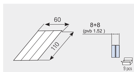
B-4009-PZ • Guarnizione ad "U" per supporto vetro 8+8 • Bottom "U" gasket for glass 8+8 • Dichtung unten für Glas 8+8
