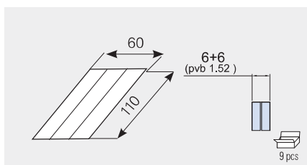
B-3507 • Guarnizione ad "U" per supporto vetro 6+6 • Bottom "U" gasket for glass 6+6 • Dichtung unten für Glas 6+6
