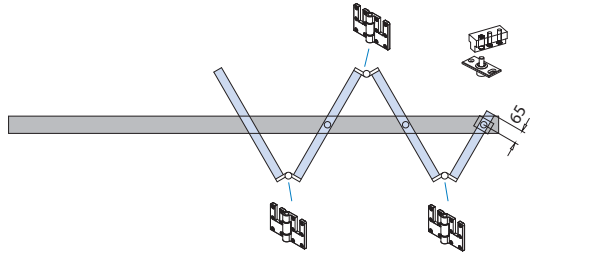
Anta libro / Folding panel/ Faltflügel
